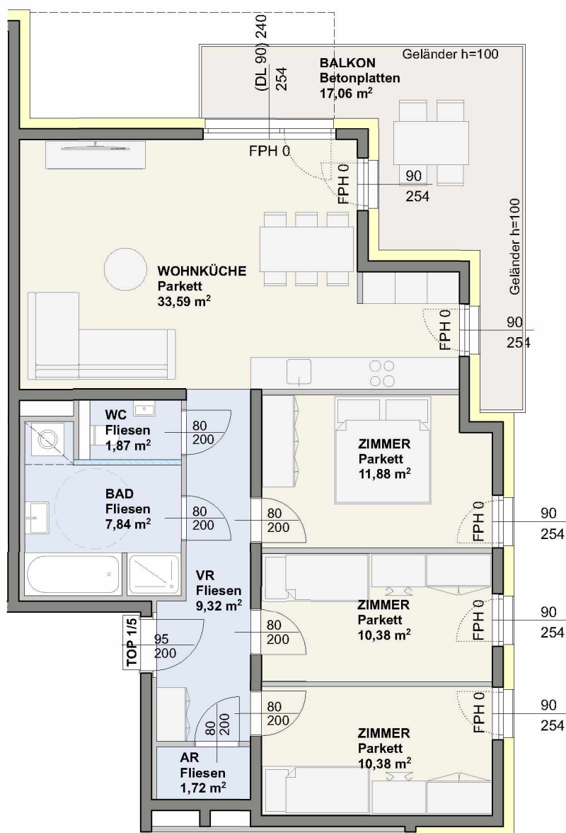
1. OBERGESCHOSS 1:100
