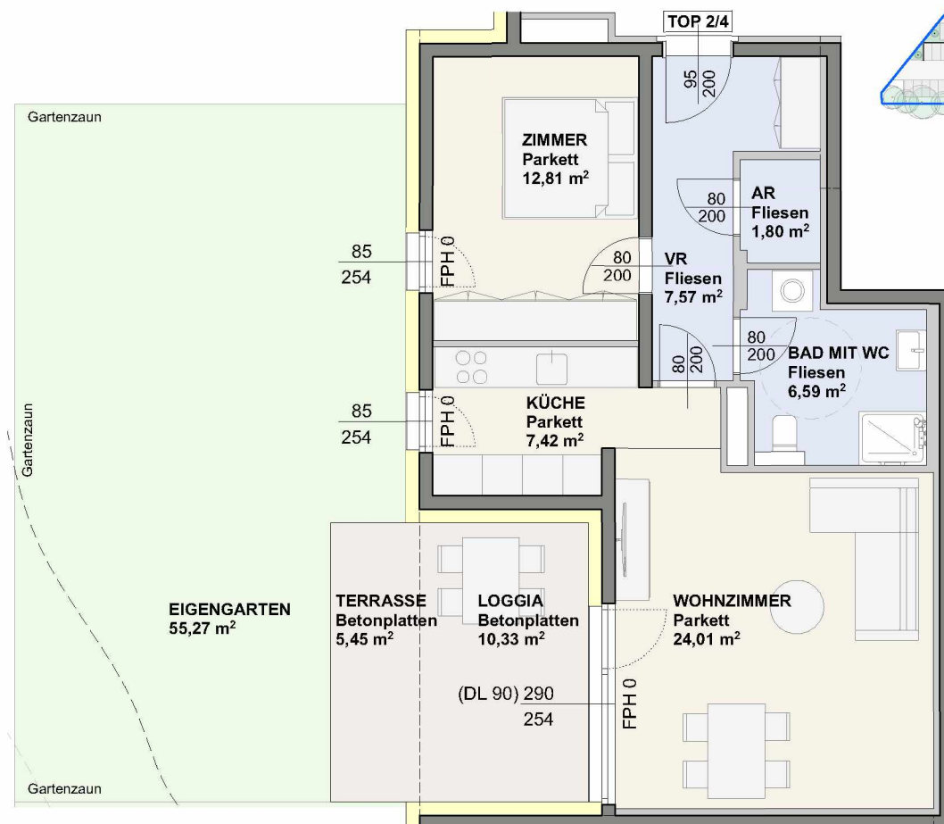
ERDGESCHOSS 1:100
