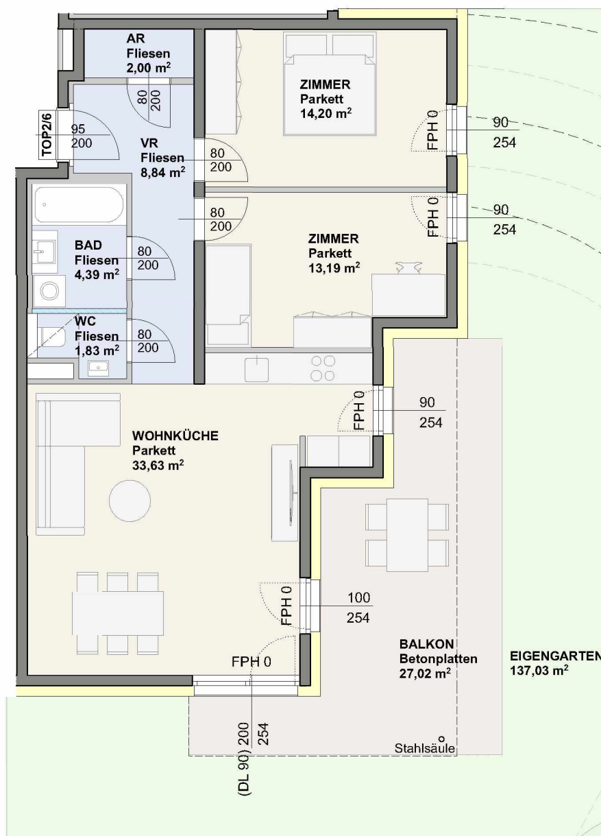
ERDGESCHOSS 1:100
