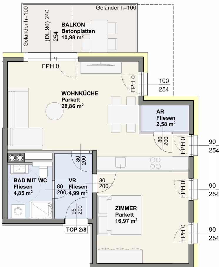
1. OBERGESCHOSS 1:100
