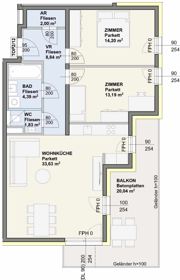
1. OBERGESCHOSS 1:100
