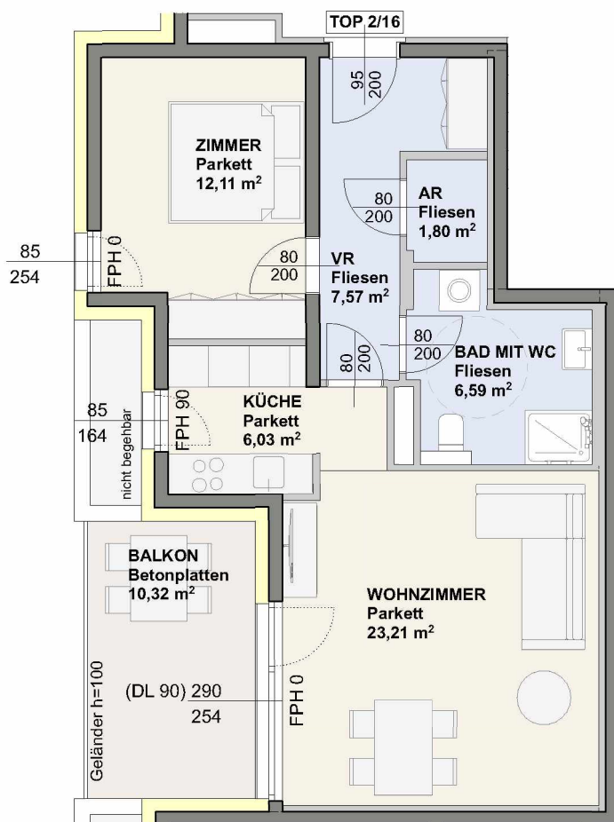
DACHGESCHOSS 1:100
