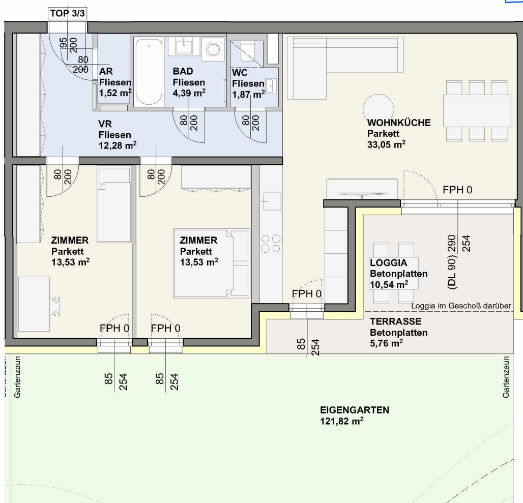
ERDGESCHOSS 1:100
