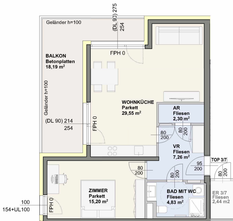
1. OBERGESCHOSS 1:100
