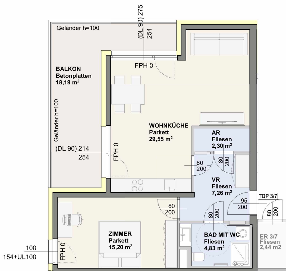
1. OBERGESCHOSS 1:100
