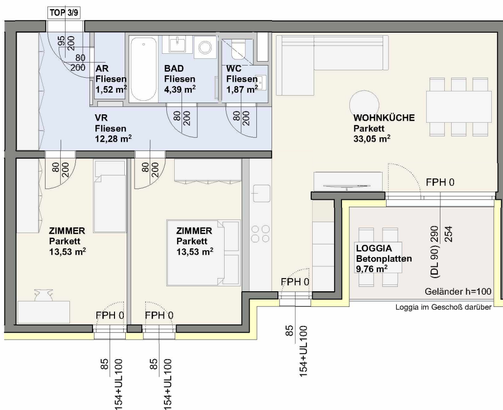
1. OBERGESCHOSS 1:100
