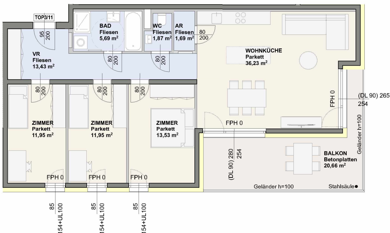
1. OBERGESCHOSS 1:100
