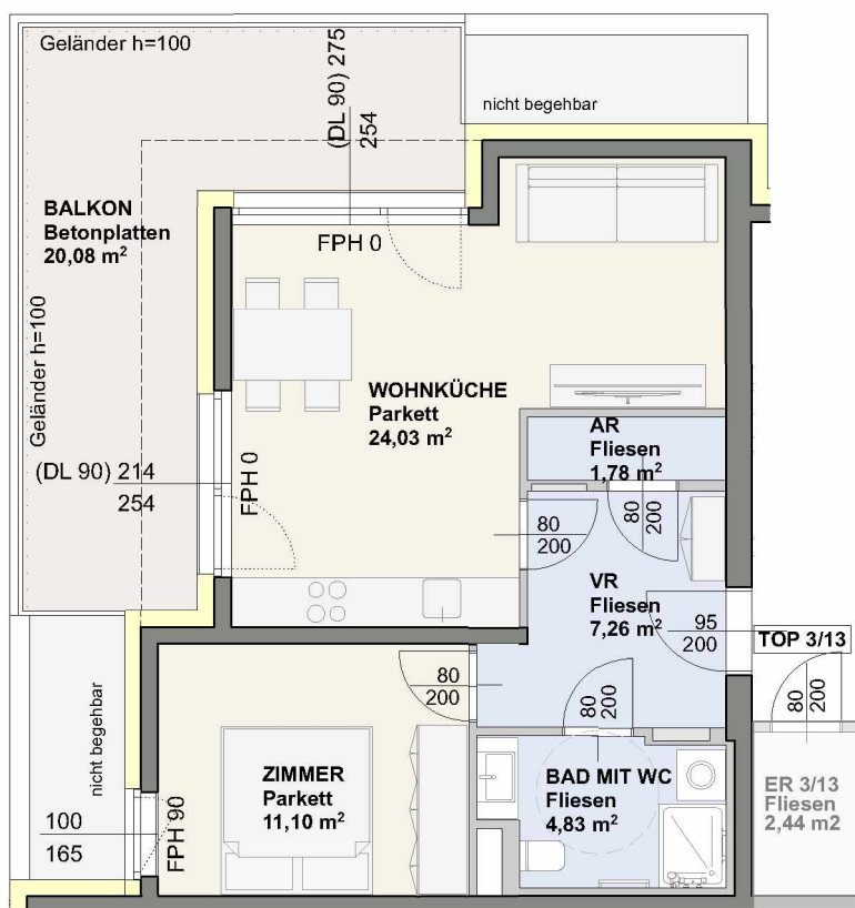
DACHGESCHOSS 1:100
