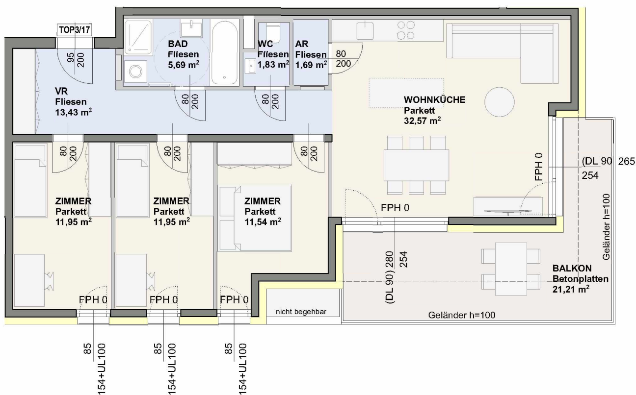
DACHGESCHOSS 1:100
