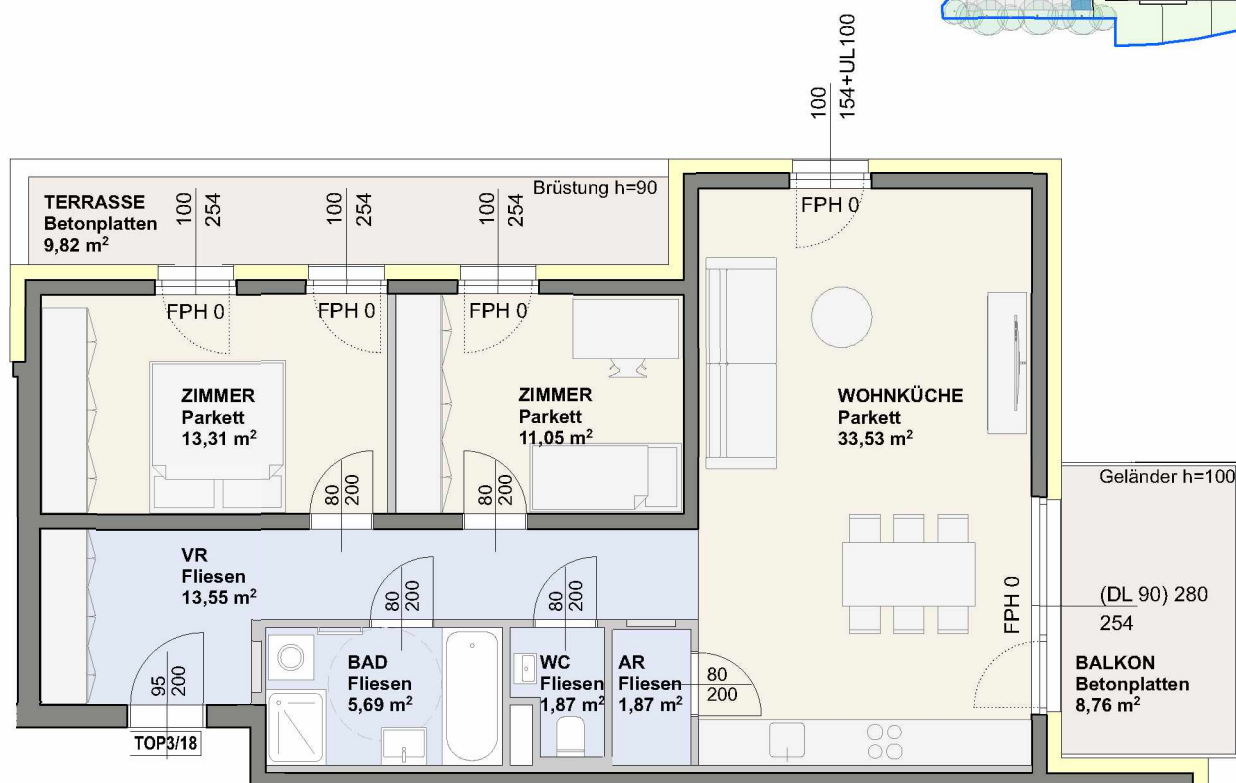
DACHGESCHOSS 1:100
