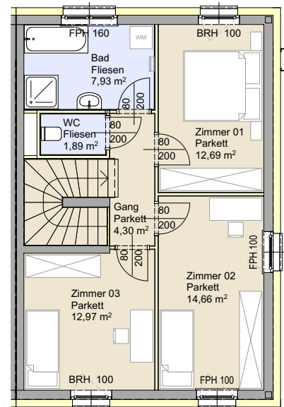
1. OBERGESCHOSS
