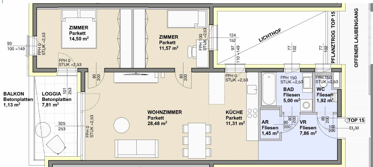
OBERGESCHOSS 1:100
